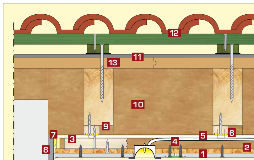
4. Unterkonstruktion mit dunklem Stift auf der „Aufdoppelung“ anzeichnen, Dampfbremsfolie an diesen Stellen antackern, anschließend einen Streifen Nageldichtband (z. B. ISOVER VARIO ANTISPIKE) aufkleben und Querlattung montieren.
