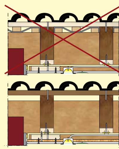
12. Abschließend die Innenverkleidung aus OSB- und Gipskartonplatten auf die Installationsebene montieren. Dabei ist darauf zu achten, dass die Platten mit versetzten Stößen angeordnet und Kreuzfugen vermieden werden.
